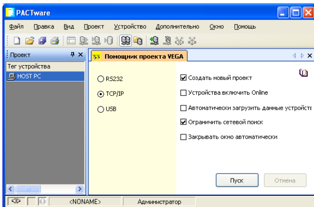
Рис. 3: Помощник проекта
