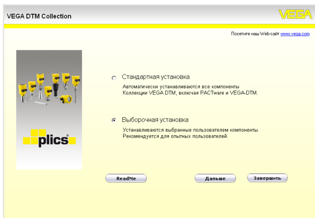
Рис. 1: Мастер установки
