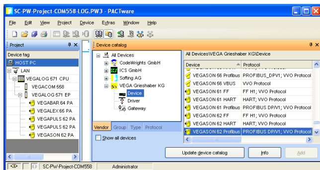
Рис. 7: Проект с VEGALOG 571 и датчиками Profibus PA
