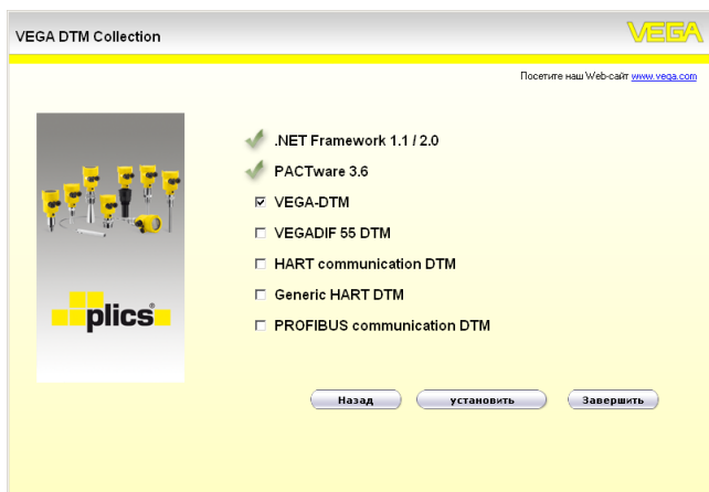
Рис. 2: Мастер установки
